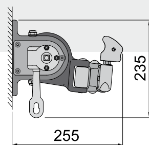
Установка на стене
