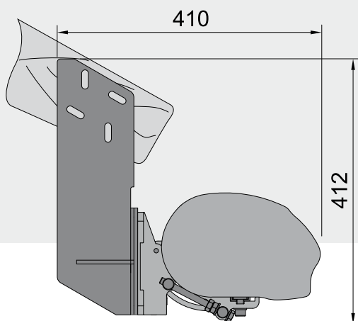
Установка на стропилах
