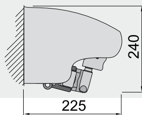
Установка на стене, вариант с защитным козырьком
