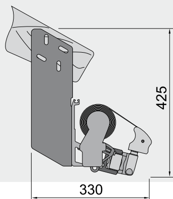
Установка на стропилах
