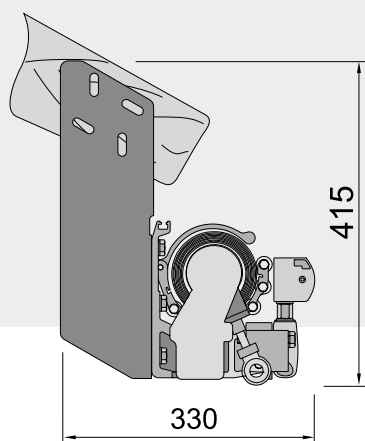
Установка на стропилах
