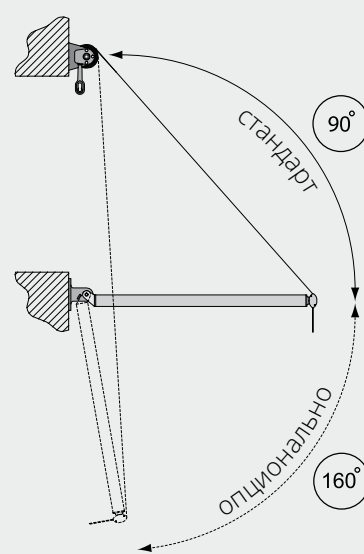
Вид сбоку, маркиза в открытом виде. Если угол превышает 90 градусов, дополнительно оплачивается ткань.
