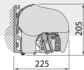
Установка на стене
