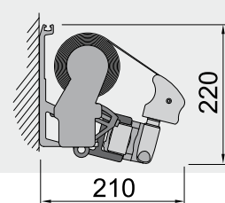
Установка на стене
