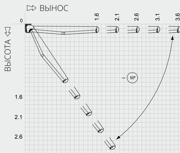
График проекции угла наклона
