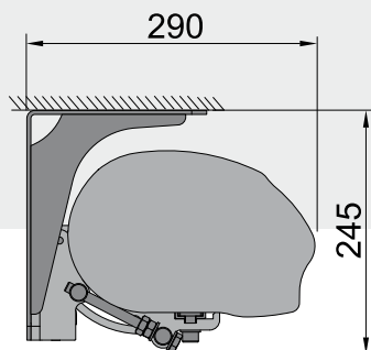
Установка на потолке
