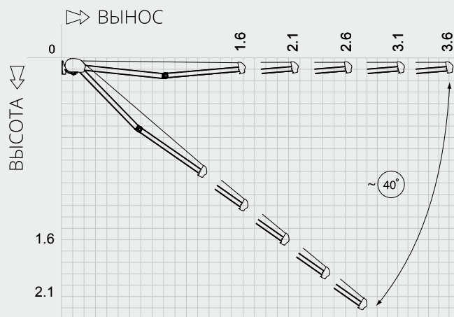
График проекции угла наклона
