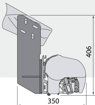
Установка на стропилах
