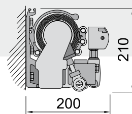
Установка на стене
