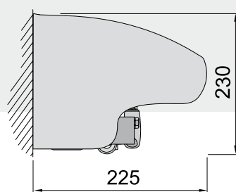
Установка на стене, вариант с защитным козырьком
