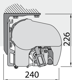
Установка на потолке
