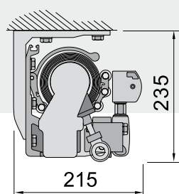
Установка на потолке
