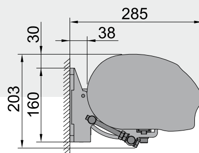
Установка на стене
